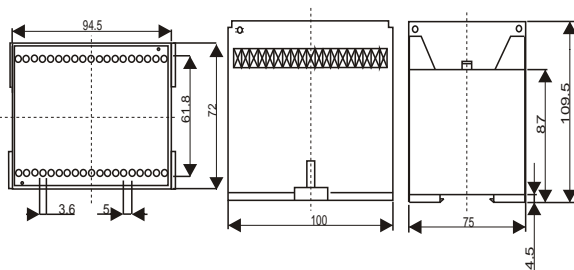
Dimensiones de la caja Case dimensions
