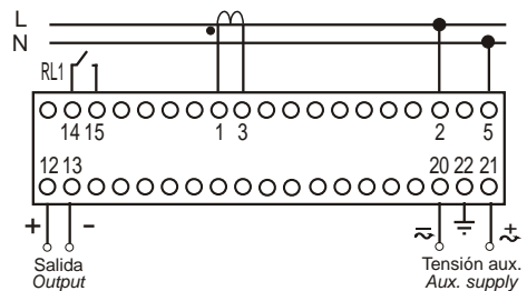
Diagrama de conexión Wiring diagram
