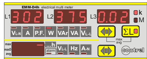
Anzeige von Blindenergiezähler 3023750.02 kVAh
