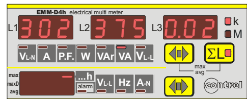
Anzeige von Scheinleistungsenergiezähler 3023750.02 kVAh
